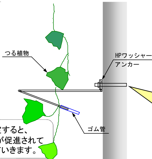
ツルキャッチャー（直付けタイプ） 側面図
