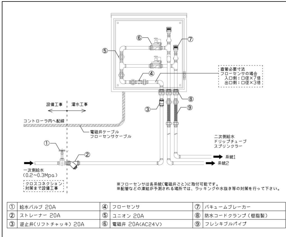
(図3) 標準配管図 壁付けタイプ
