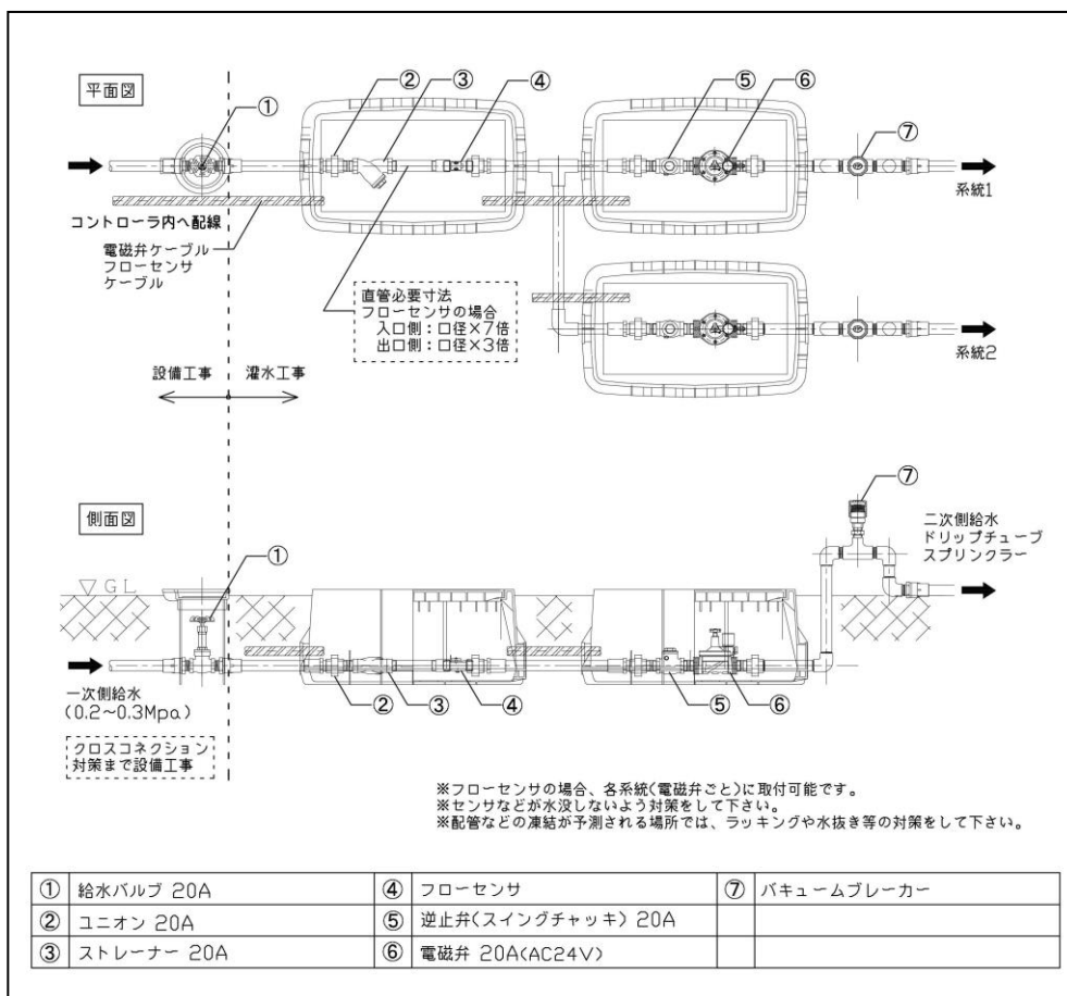
(図4) 標準配管図 埋設タイプ
