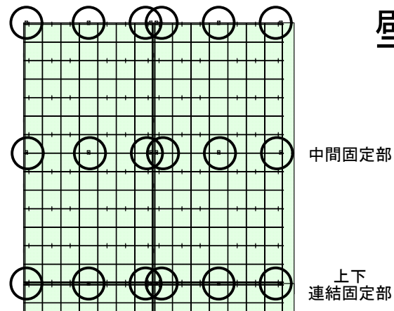
固定金具の標準位置 (パネル縦づかいの場合)
